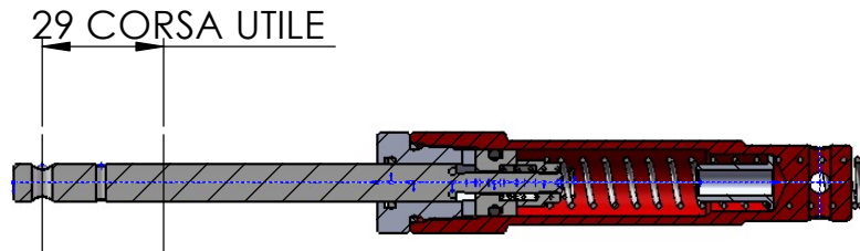
SEZIONE A-A
