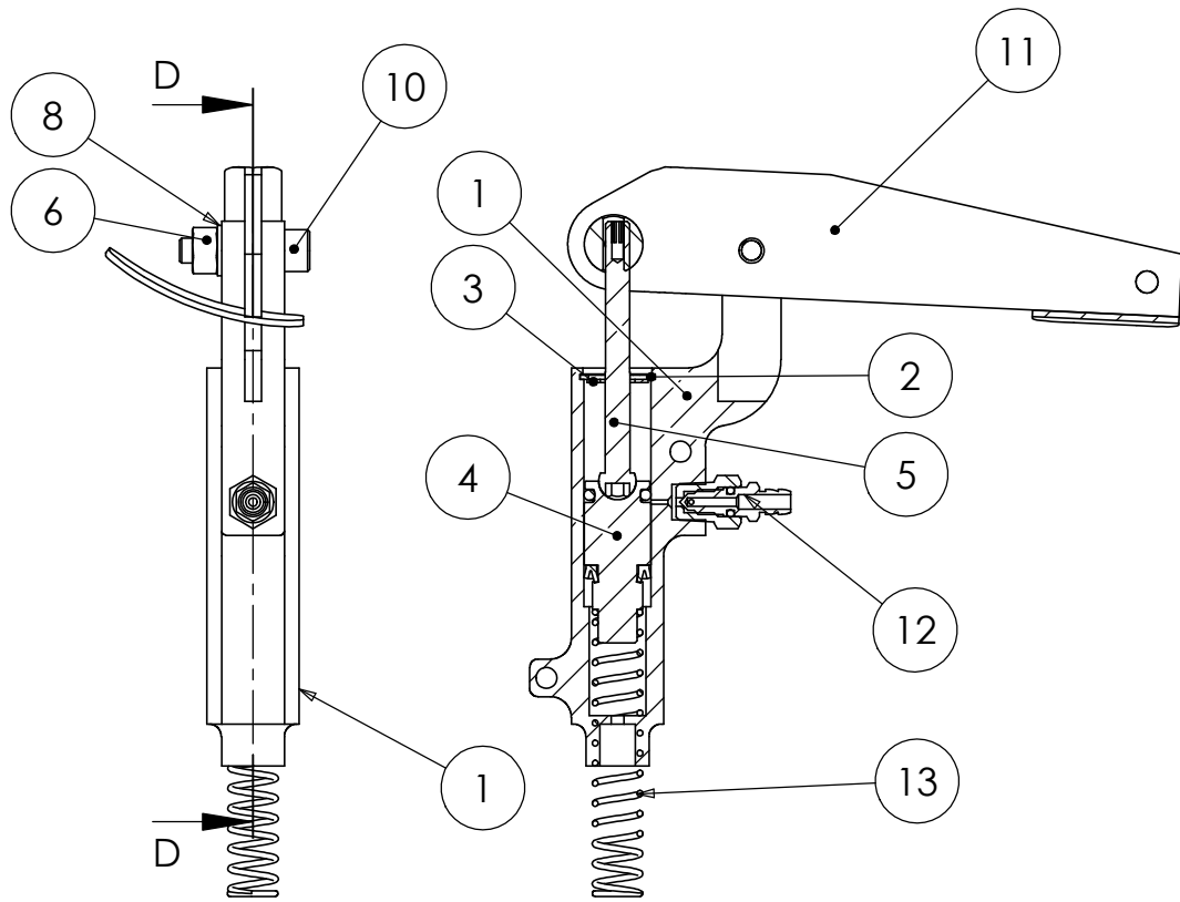
SEZIONE D-D
