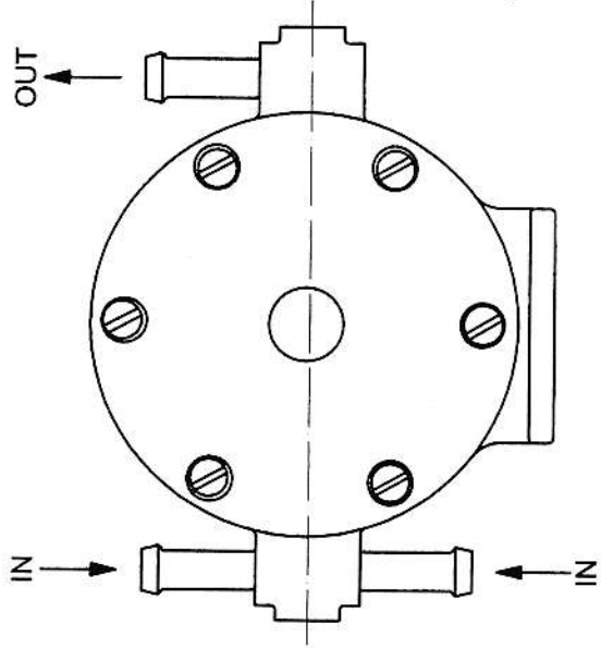
VISTA DALL'ALTO
