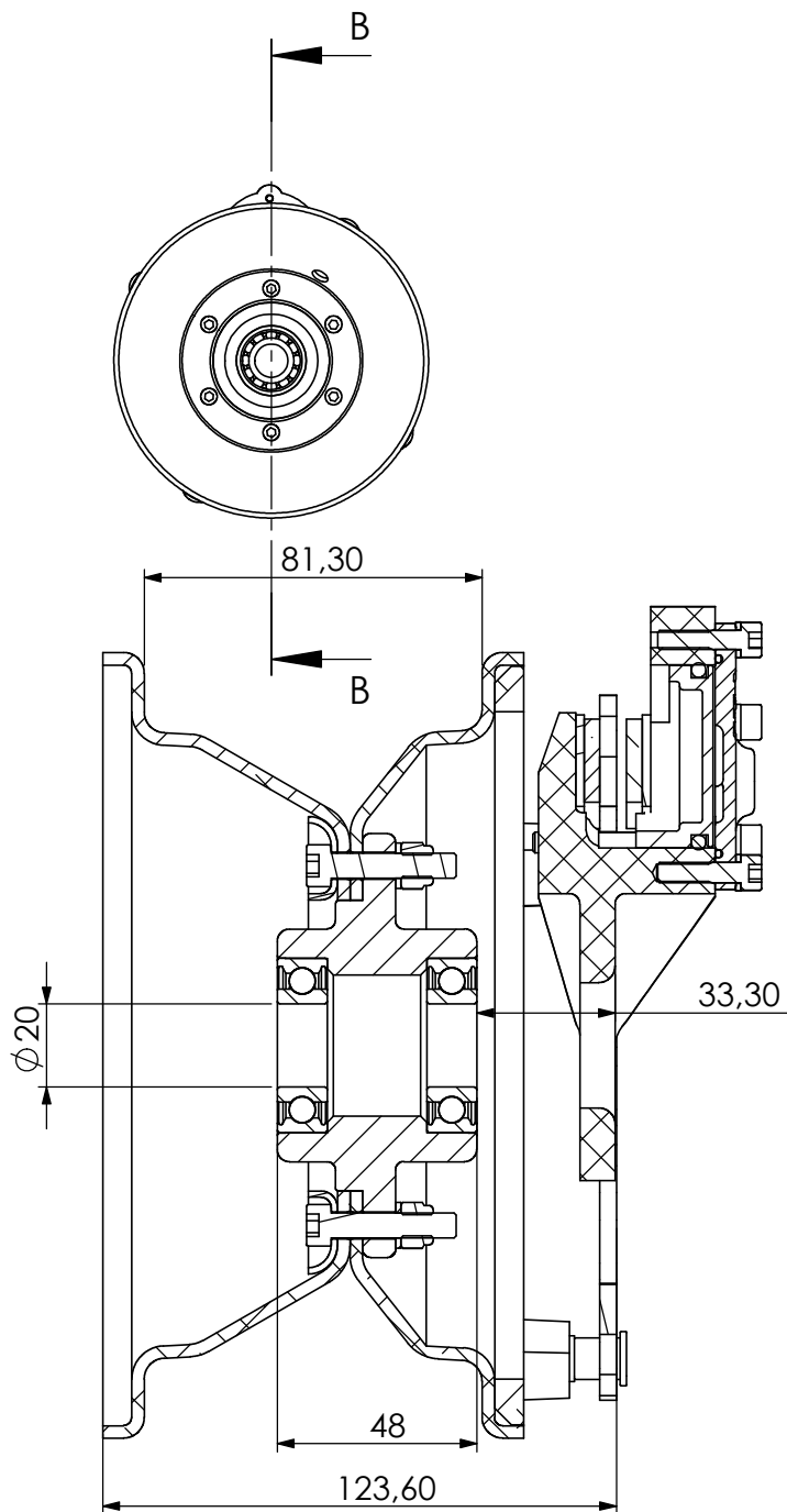
SEZIONE B-B
