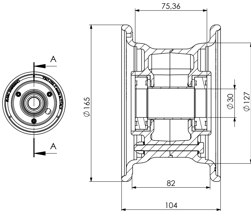
SEZIONE A-A SCALA 1 : 2
