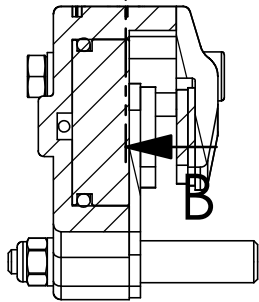
SEZIONE B-B SCALA 1 : 2
